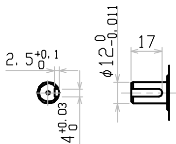
シャフト詳細図
